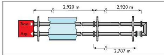
PANRAD FRA – dl.6m, z trubek dl.3m
