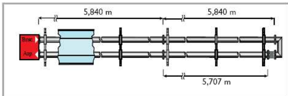
PANRAD FRC – dl.12m, z trubek dl. 6m
