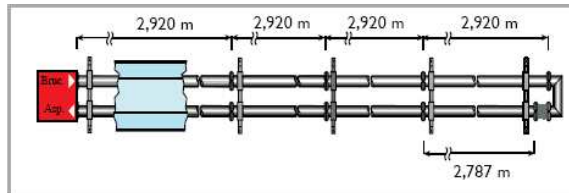
PANRAD FC – dl.12m, z trubek dl. 3m
